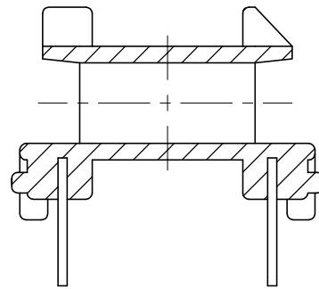
SEC. A-A
