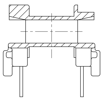
SEC. A-A
