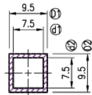
A-A Section
